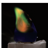
「青色折り紙の炎色反応」 石川 智久
